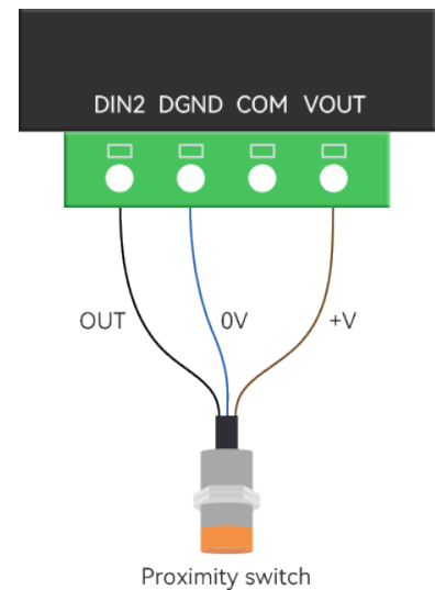
DI (NPN/PNP) Wiring Diagram
