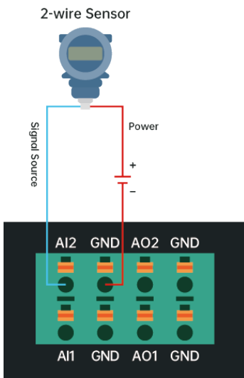
AI (2-wire) Wiring Diagram
