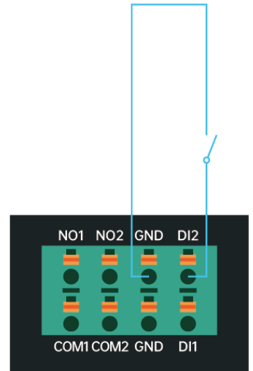
DI Wiring Diagram
