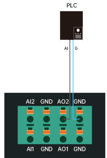
AO Wiring Diagram
