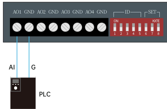
AO Wiring Diagram
